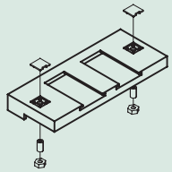
Conjunto cortavientos ALAS 70 Ref. 2202011000
