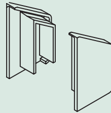
Conjunto tapa remate 01203 Ref. 2406403000
